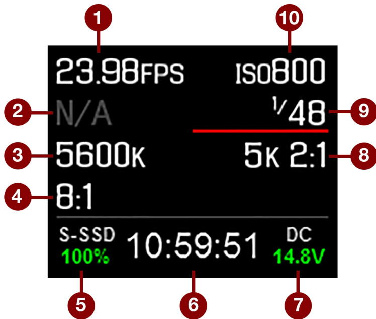
图：DSMC2 SIDEKICK OLED( 本机模式)
