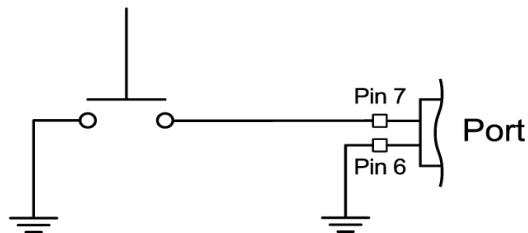
图：触点闭合式触发器按钮电路图
