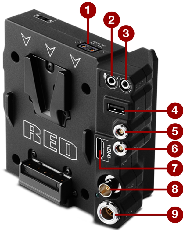
图：DSMC2 V-Lock I/O 扩展器
