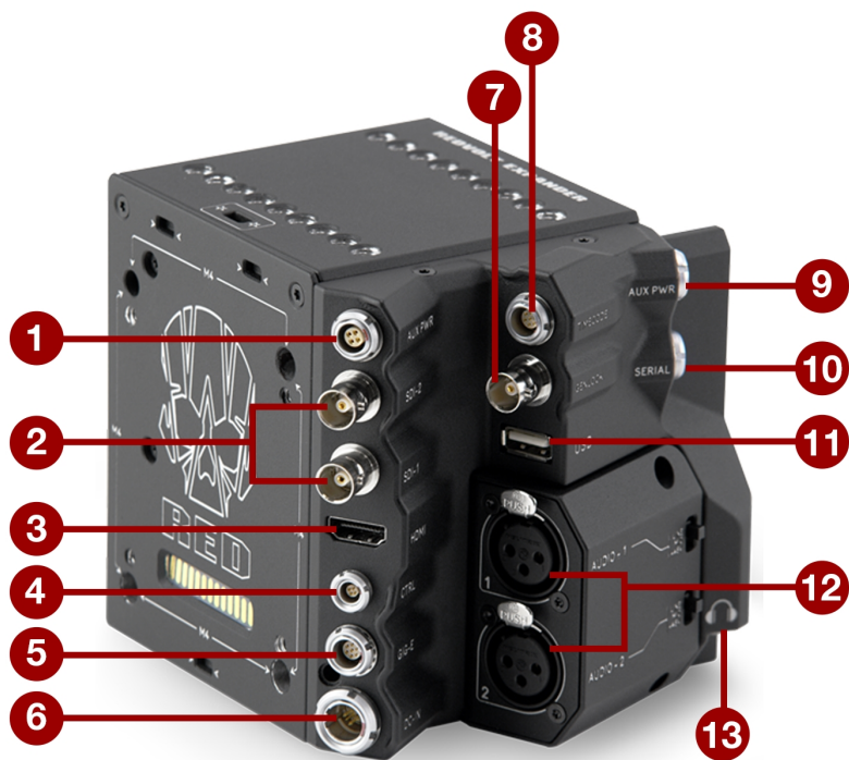
图：DSMC2 REDVOLT 扩展器
