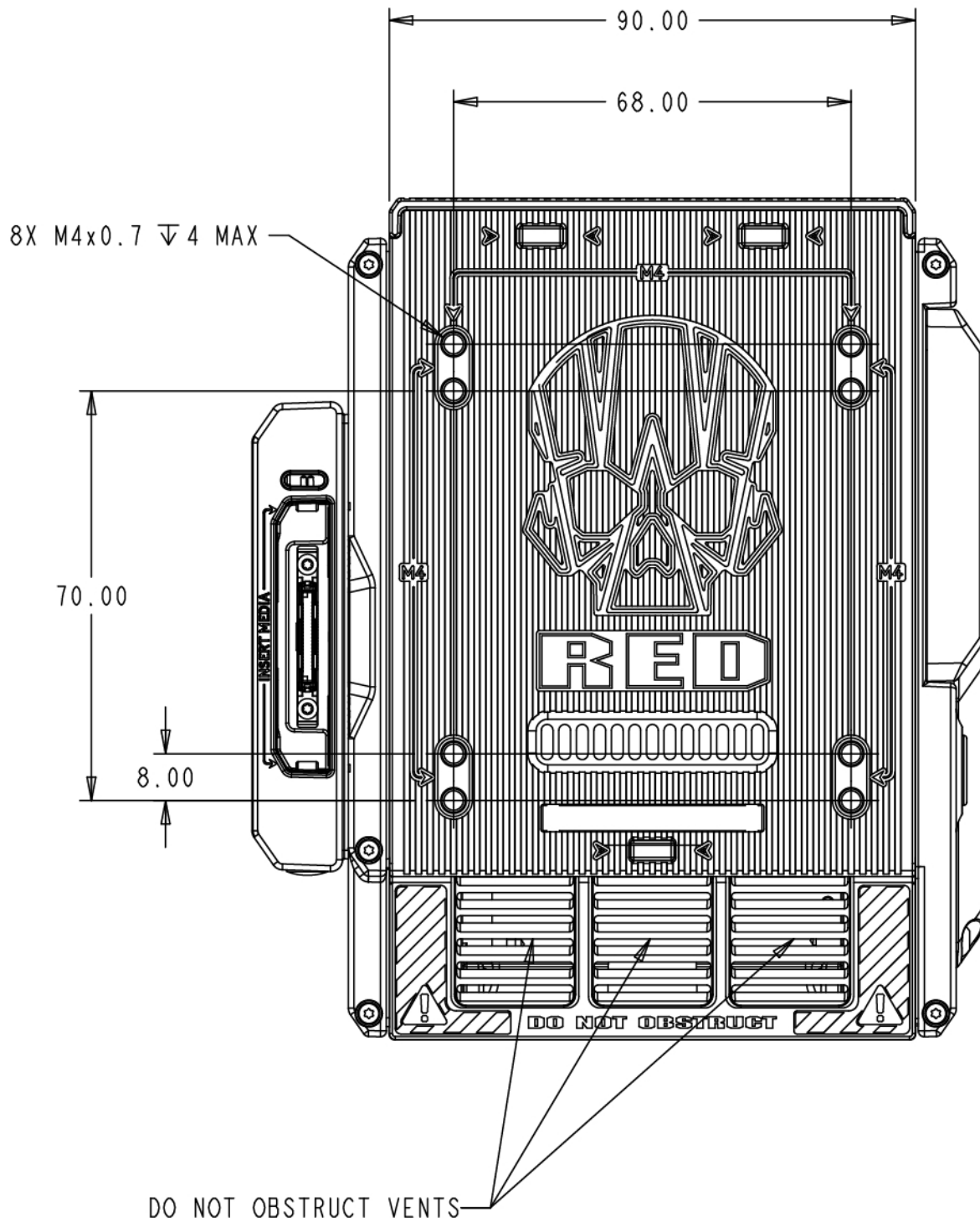
图 : RAVEN Back View
