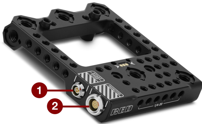
图：DSMC2 战术顶板
