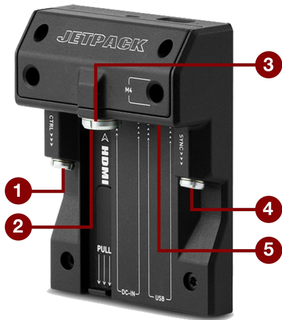
图：DSMC2 Jetpack 扩展器
