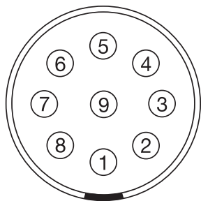
图：GIG-E连接器的正面( 观察摄影机)
